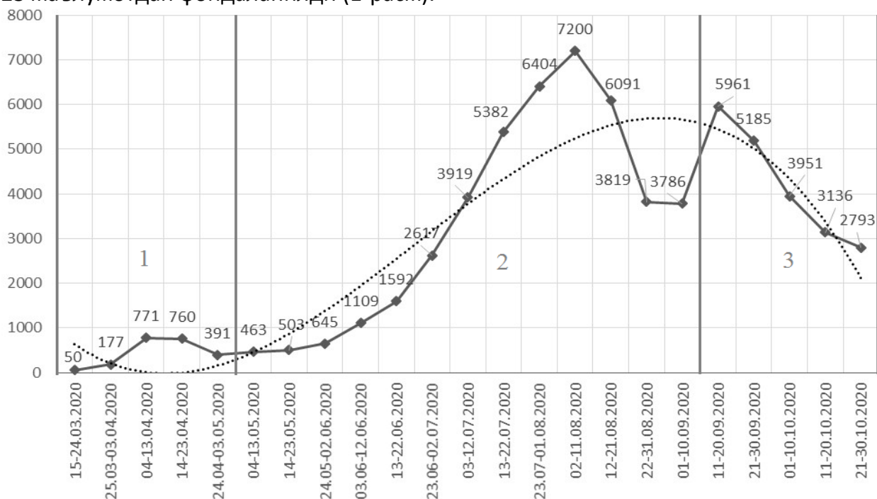
1-расм. 2020 йилнинг 15 мартдан 30 октябригача бўлган муддатда коронавирус касаллигига чалинган беморлар сонининг динамикаси, киши ҳисобида.
