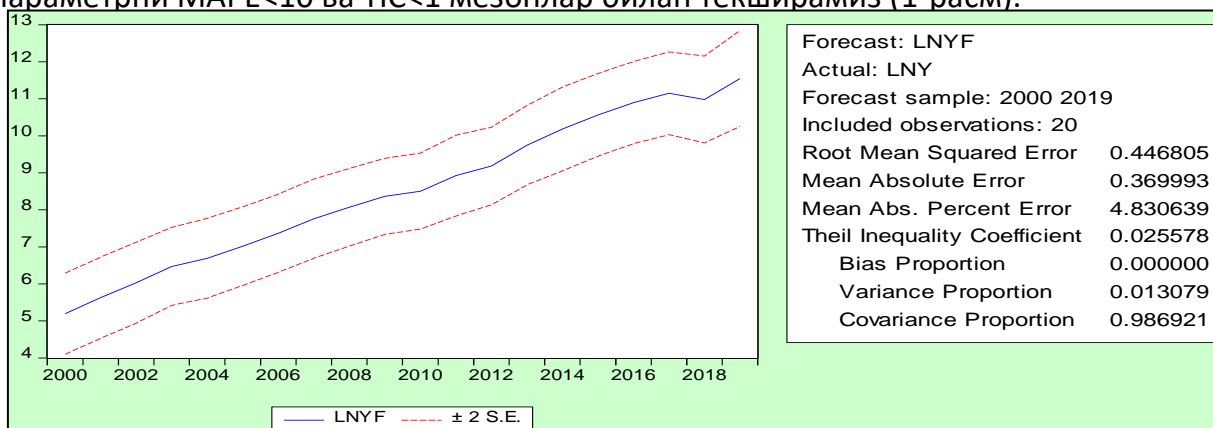
1-расм. Ўзгарувчининг ретроспектив прогноз сифатини баҳолаш 3
